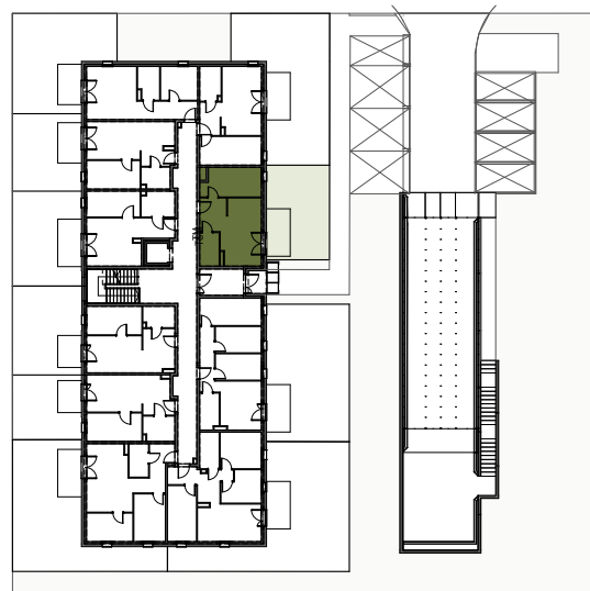
RZUT PARTERU
