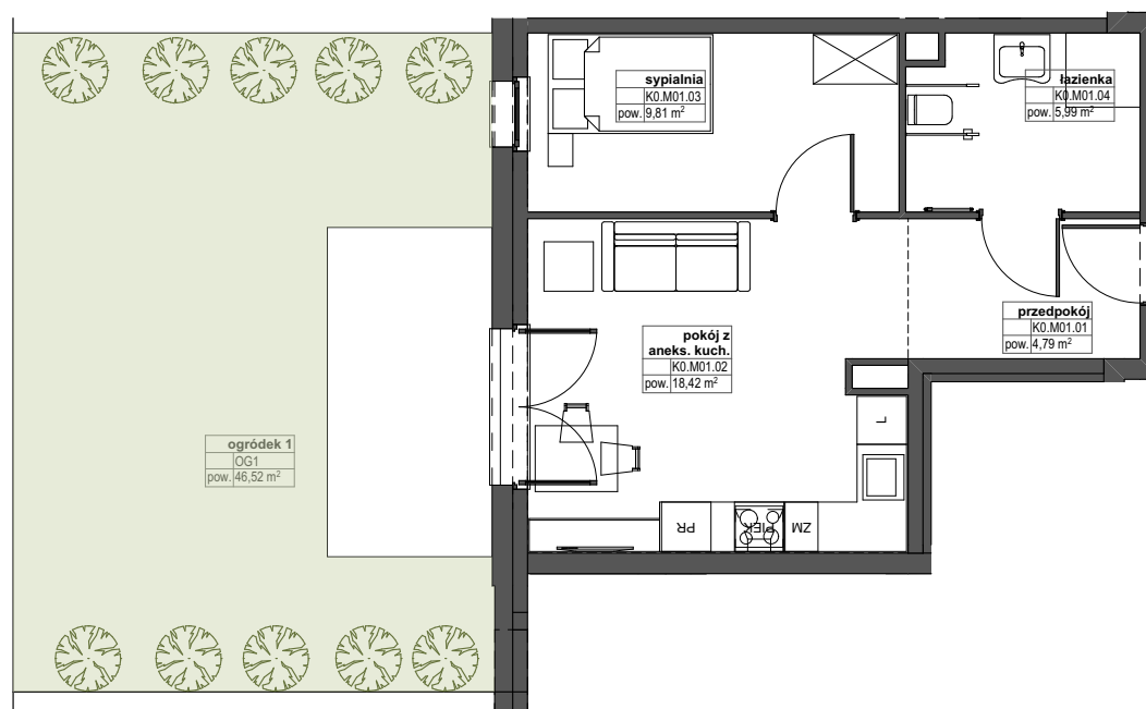
RZUT PARTERU
