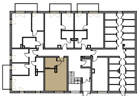
RZUT PARTERU BUDYNEK B
